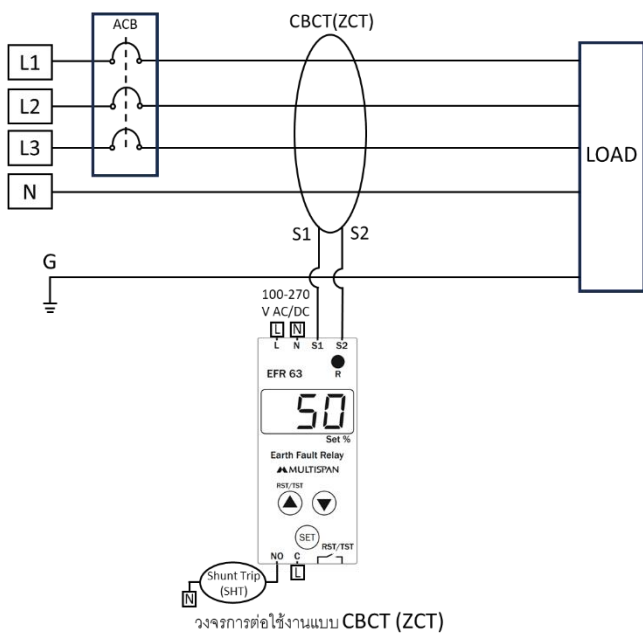
วงจรการต่อใช้งานแบบ CBCT (ZCT)
