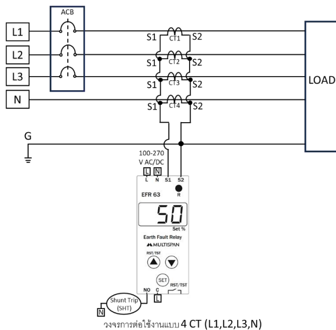
วงจรการต่อใช้งานแบบ 4 CT (L1,L2,L3,N)
