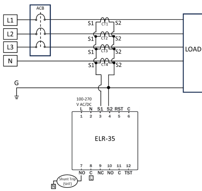
วงจรการใช้งานแบบ 4 CT (L1,L2,L3,N)
