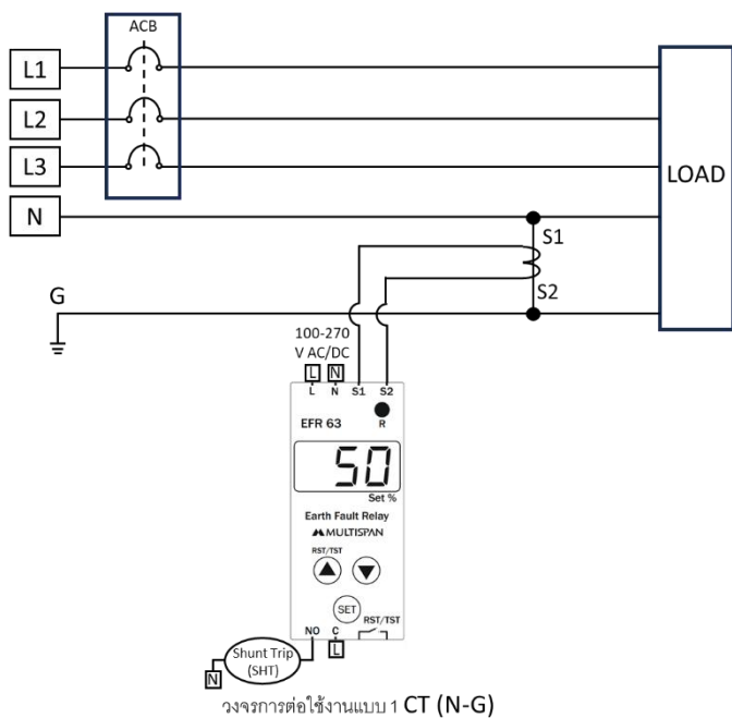
วงจรการต่อใช้งานแบบ 1 CT (N-G)
